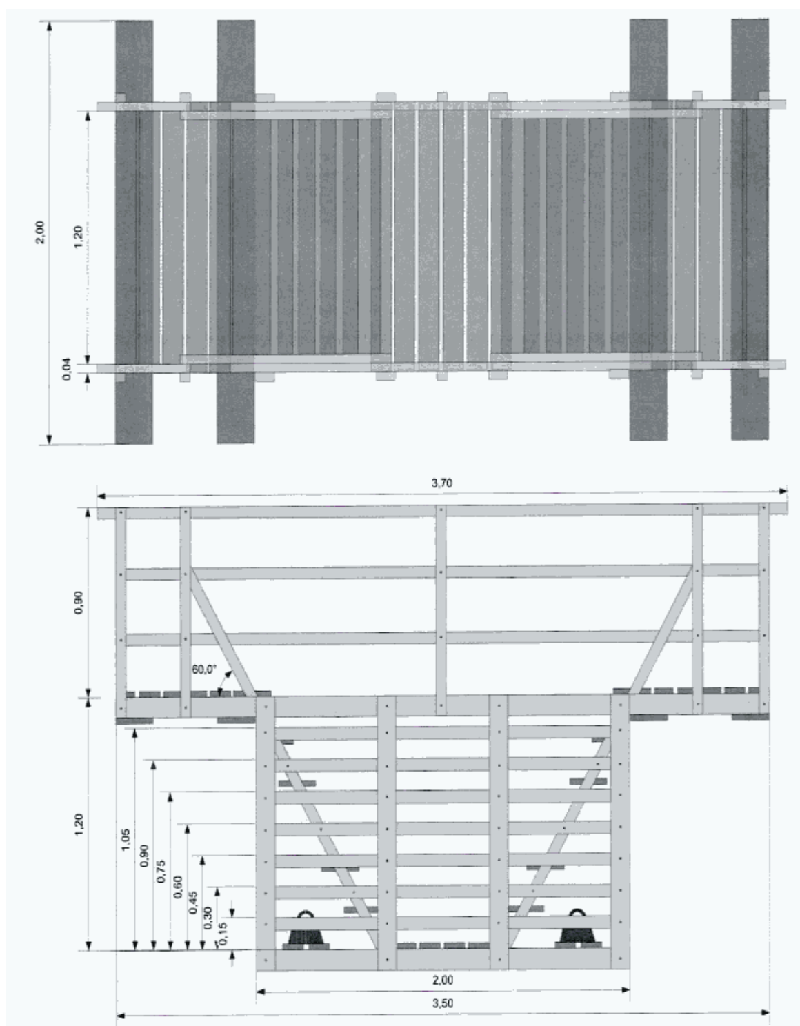
Чертеж конструкций мостков для Крещенских купаний на водных объектах (вариант 1)
