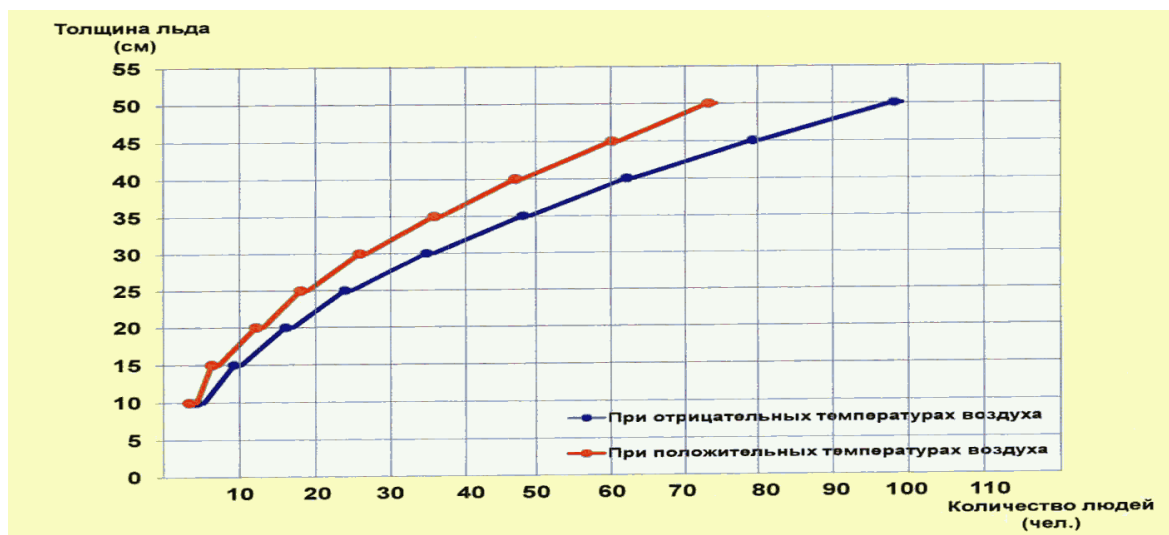
Рис. 1 График зависимости максимального допустимого количества людей на льду площадью 100 м 2 (10 x 10) от толщины льда
